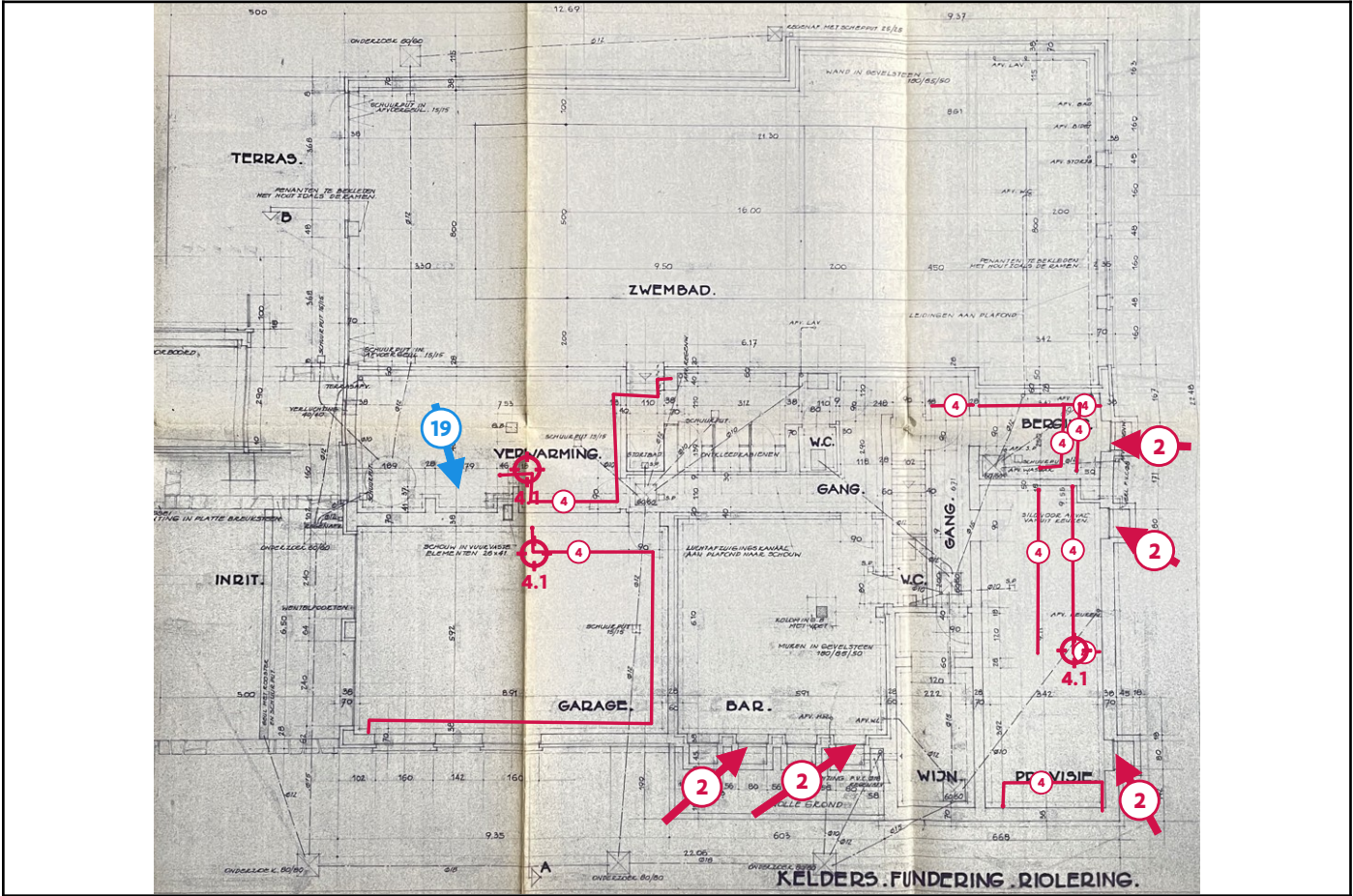
Legende van plan 1.4: Kelderplan Leterweg 65 te Bilzen
