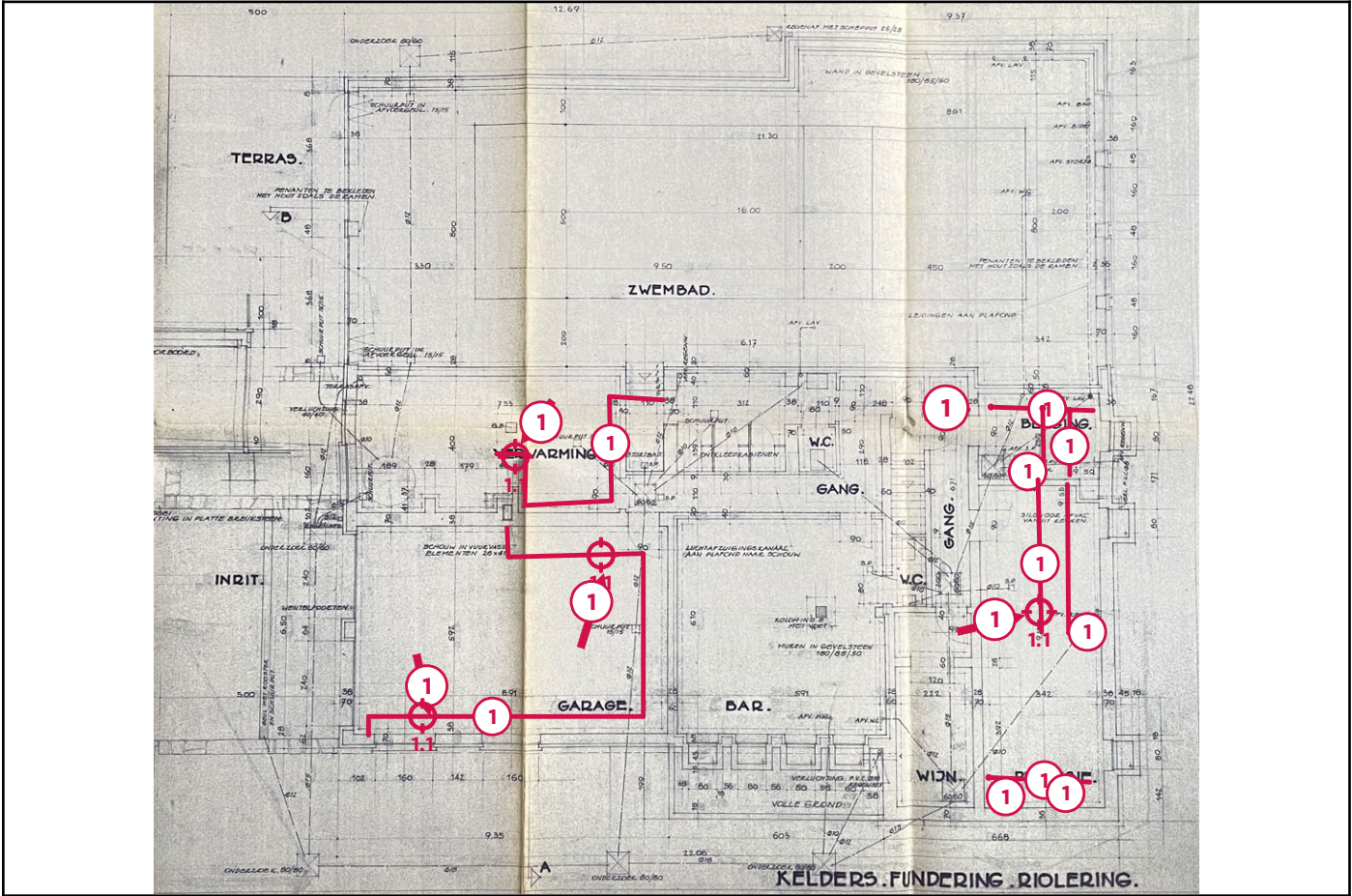
Legende van plan 1.8: Kelderplan Leterweg 65 te Bilzen
