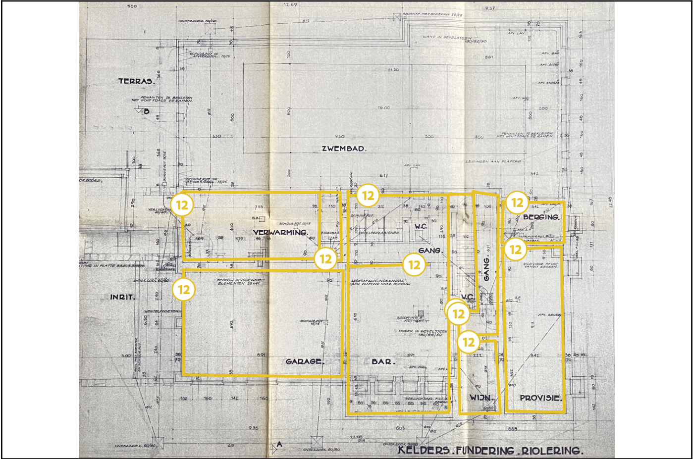
Legende van plan 1.5: Kelderplan Leterweg 65 te Bilzen
